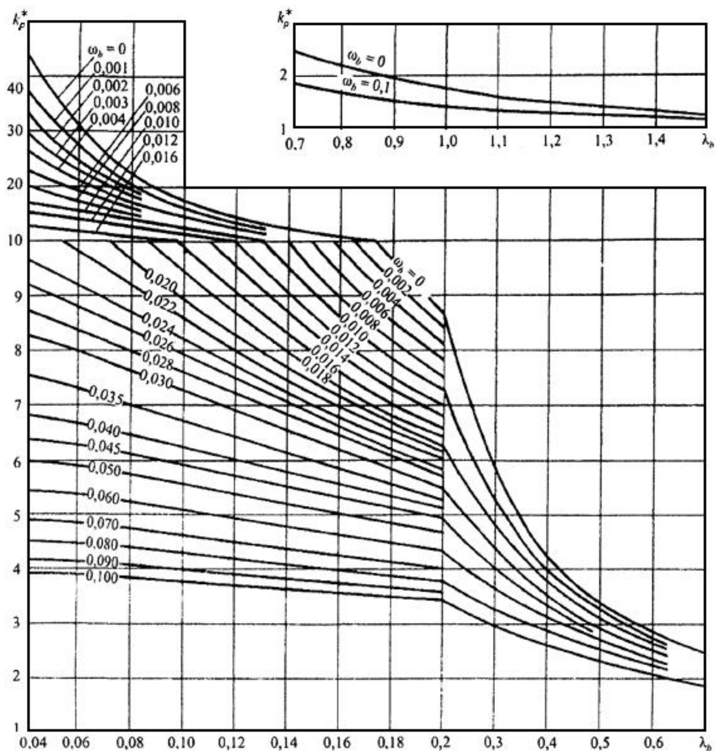
Рисунок 1 - График для определения значений коэффициента k_p^*
