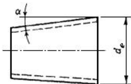
Рисунок А.2 - Концентрический переход
