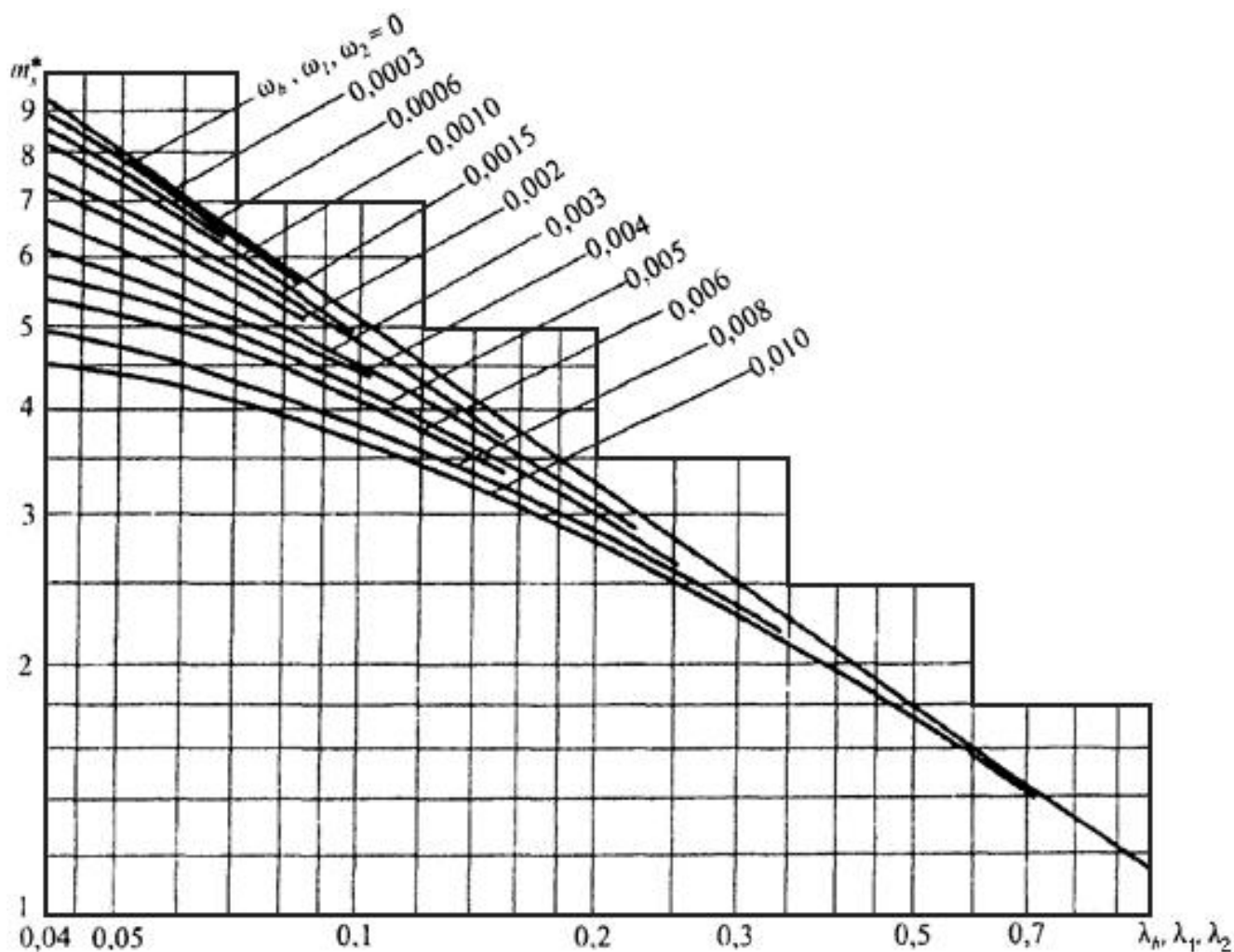
Рисунок 2 - График для определения значений коэффициента m_s^*
