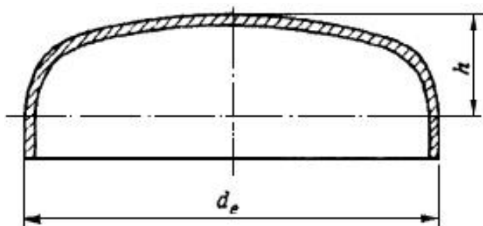
Рисунок А.3 - Заглушка эллиптическая
